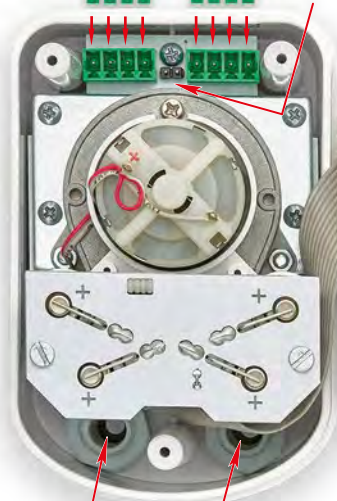
Фото 6. Электропривод управления шаровым краном со снятой крышкой
