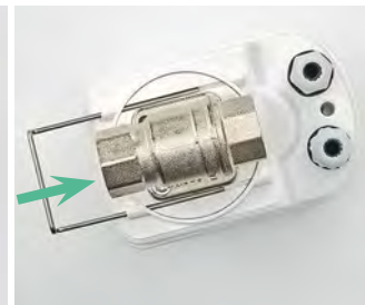
Фото 26. Крепление электропривода к шаровому крану с помощью металлической скобы
