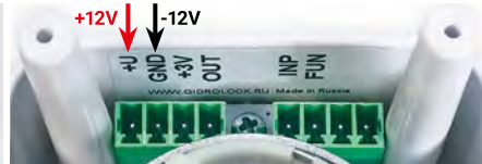
Фото 20. Клеммы разъема электропривода для подключения внешнего блока питания +12 В, проводного выключателя, объединения в систему нескольких шаровых электроприводов
