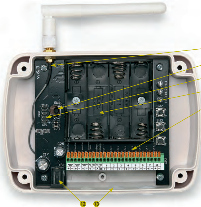
Фото 4. Блок управления GIDROLOCK Wi-Fi V5 со снятой фронтальной крышкой
