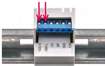
Фото 3. Подключение к сети 220 Вольт.
