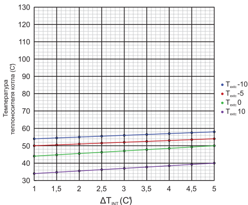
Рис.12 Тепловая кривая с K_{comp}=2 .
