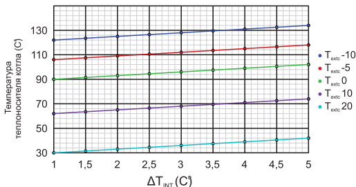
Рис.9 Тепловая кривая с K_{comp}=6 «значение по умолчанию».
