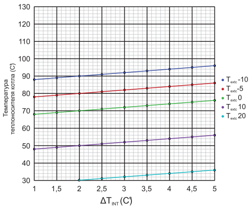
Рис.11 Тепловая кривая с K_{comp}=4 .
