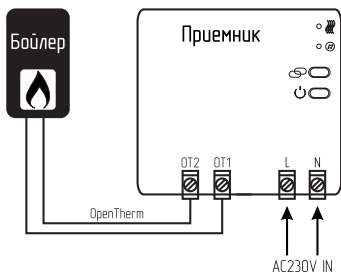
Рис.7 Схема подключения котла к терморегулятору по цифровой шине OpenTherm.
