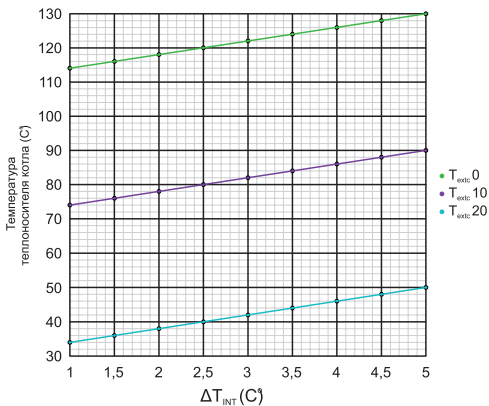
Рис.10 Тепловая кривая с K_{comp}=8 .
