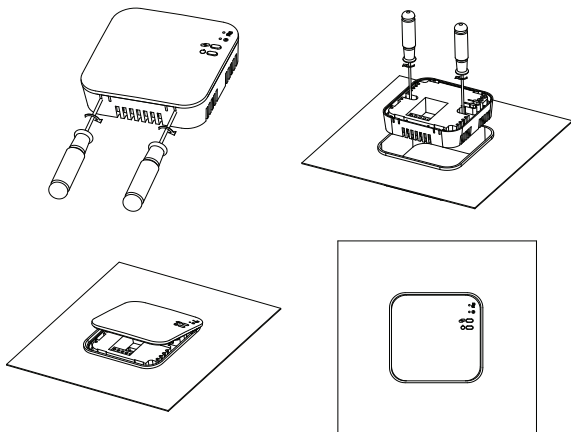
Рис.5 Установка приемника терморегуляторов Smart Link Wi-Fi OT на стену.
